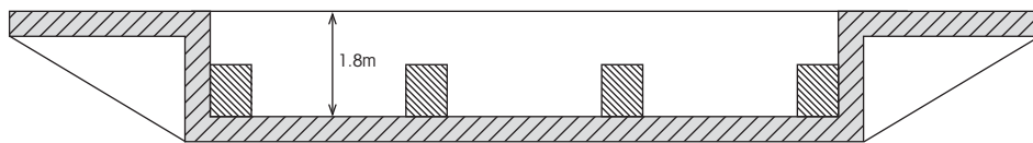
深基坑基础(等截面梁的秤台)
